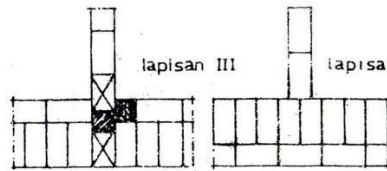
PERTEMUAN TEGAK DARI 1/2 + 1 1/2 BATA
