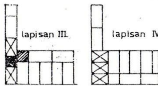
SUDUT TEGAK DARI 1/2 + 1 1/2 BATA
