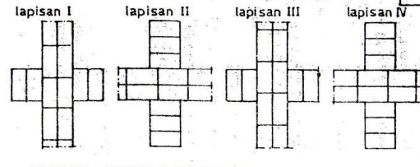
SILANGAN TEGAK DARI TEMBOK 1 BATA
