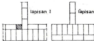
SILANGAN TEGAK DARI TEMBOK 1 BATA
