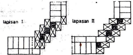
PERTEMUAN TEGAK DARI TEMBOK 1/2 + 1 BATA
