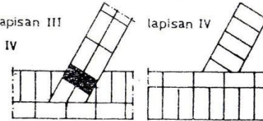
PERTEMUAN SERONG DARI 1 + 1/2 BATA
