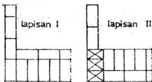
SILANGAN TEGAK DARI TEMBOK 1/2 + 1 BATA
