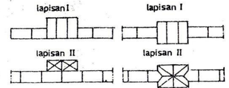
TIANG2 TEMBOK DARI 1 BATA
