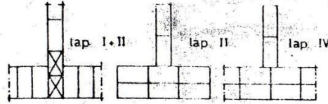
PERTEMUAN TEGAK DARI TEMBOK 1/2 + 1 BATA
